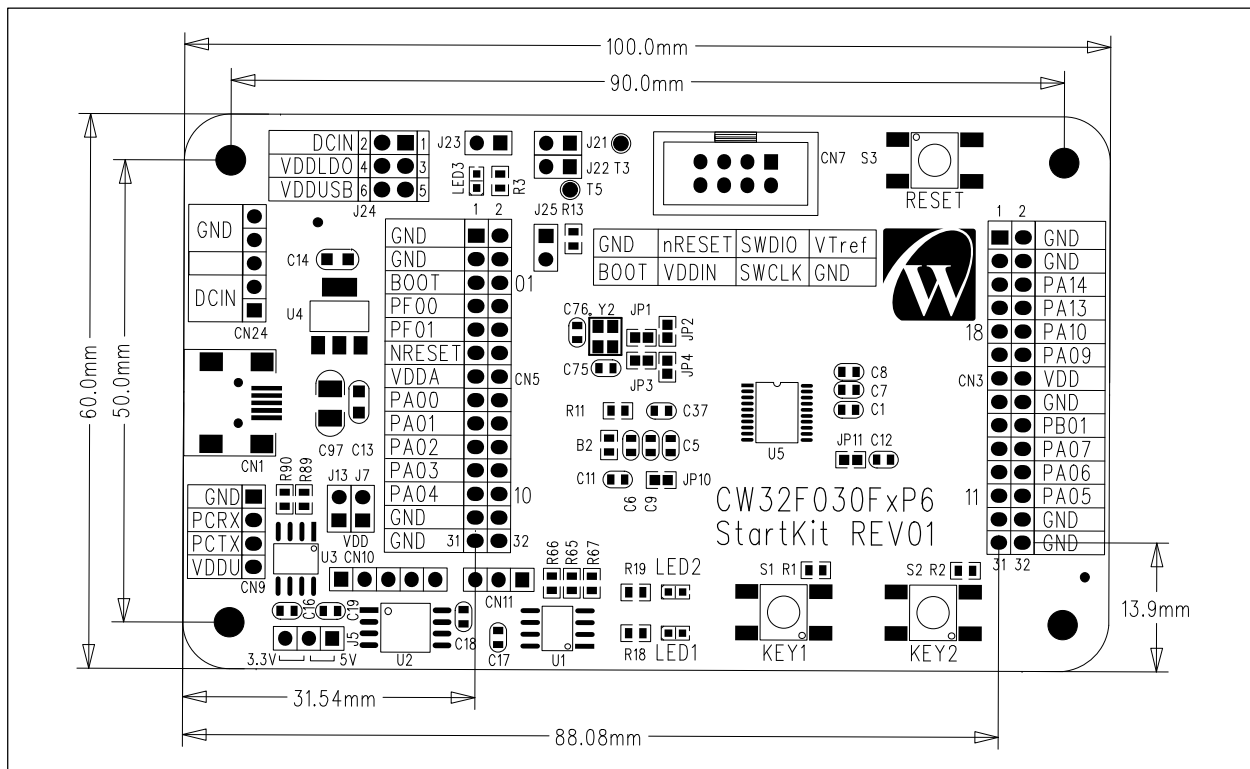
图 6-2 CW32F030FxPx StartKit 机械尺寸
