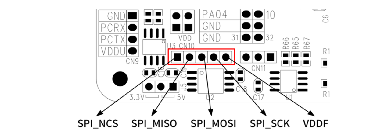
图 6-5 CN10 引脚定义
