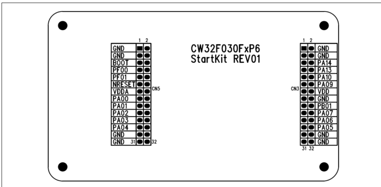
图 6-4 扩展接口布局
