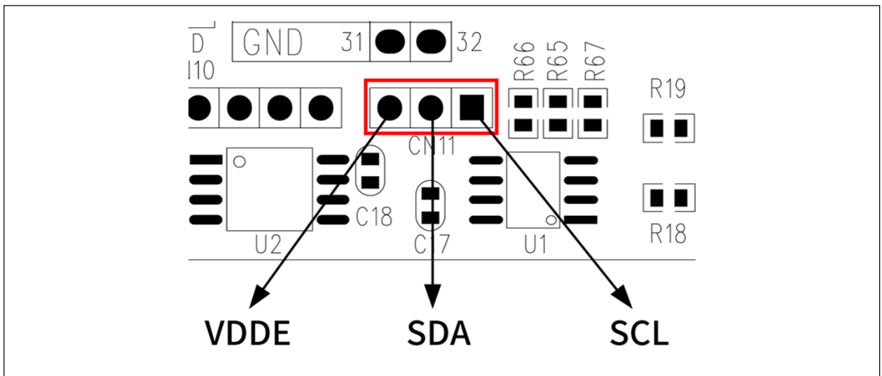
图 6-6 CN11 引脚定义
