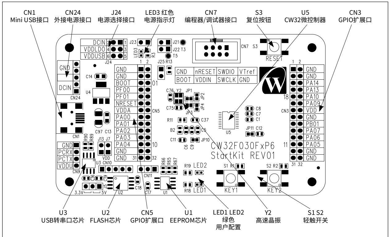
图 6-1 顶层器件布局
