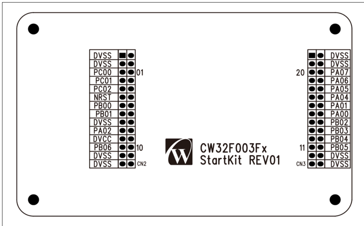
图 6-4 扩展接口布局
