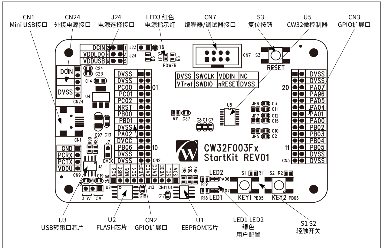
图 6-1 顶层器件布局
