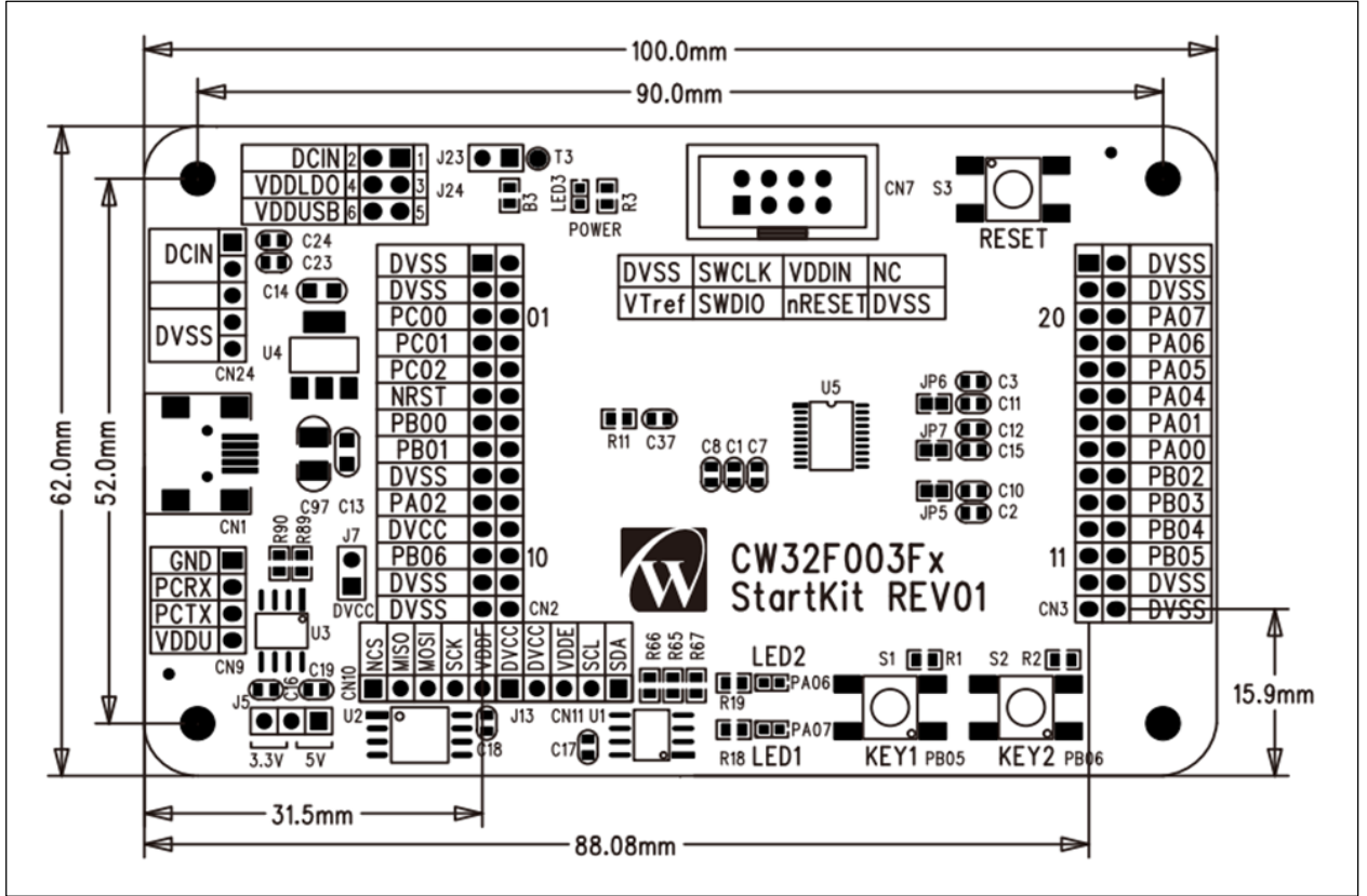
图 6-2 CW32F003FxFx StartKit 机械尺寸
